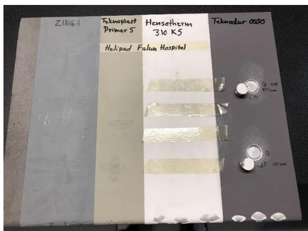
Het coatingsysteem voor de draagbalken en dwarsliggers op de 4 parkeerverdiepingen onder het FALUN Hospital Helipad.
